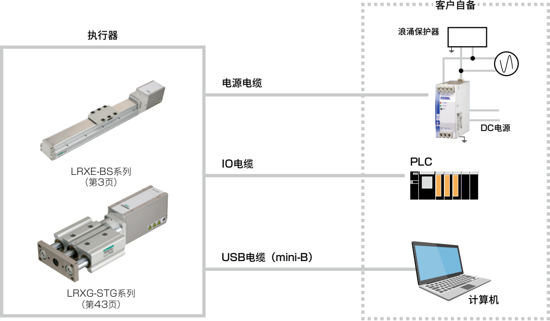
系统构成图
