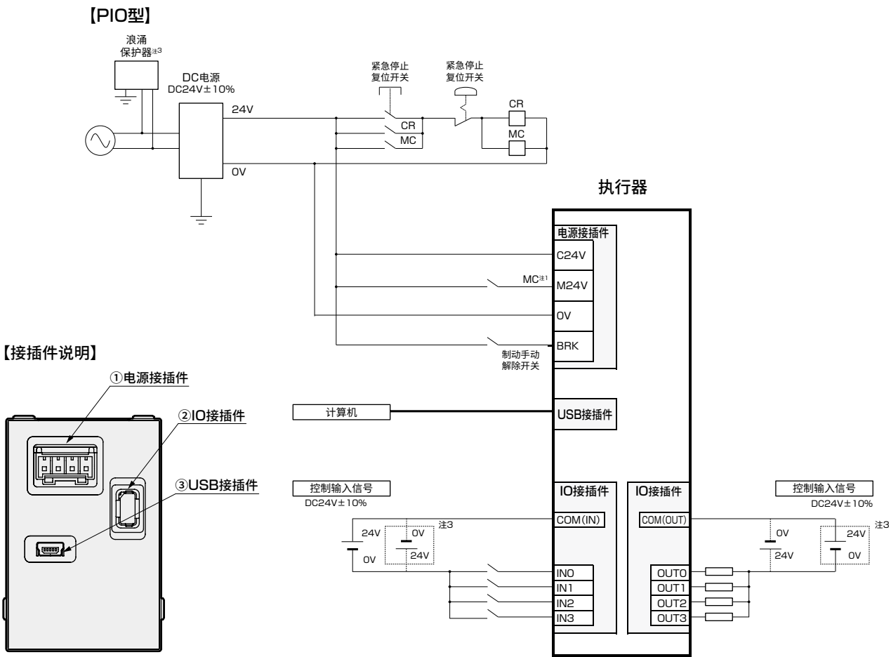
并行I/O(PIO)连接图
