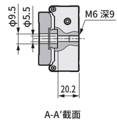
A-A'截面
