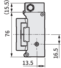
接插件伸出方向L(左侧面)时
