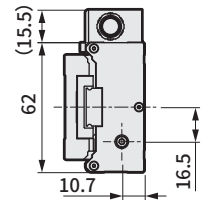
接插件伸出方向L(左侧面)时
