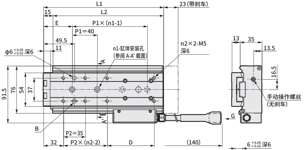
接插件伸出方向L(左侧面)时
