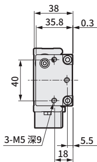
接插件伸出方向R(右侧面)V规格时
