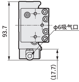
接插件伸出方向R(右侧面)V规格时
