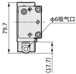
接插件伸出方向R(右侧面)V规格时
