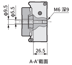
A-A'截面
