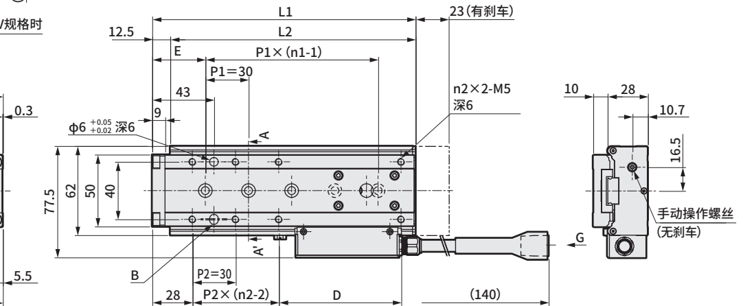
接插件伸出方向L(左侧面)时
