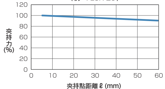
夾持力和夾持點距離 (例: FLSH-20)
