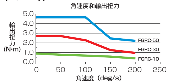
【DC24V時】
