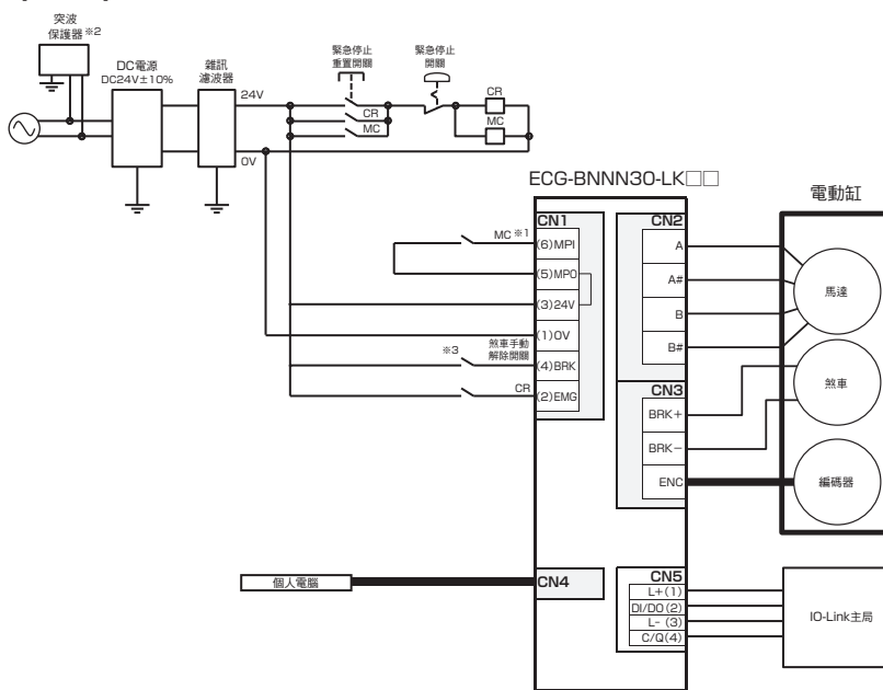
【IO-Link型】
