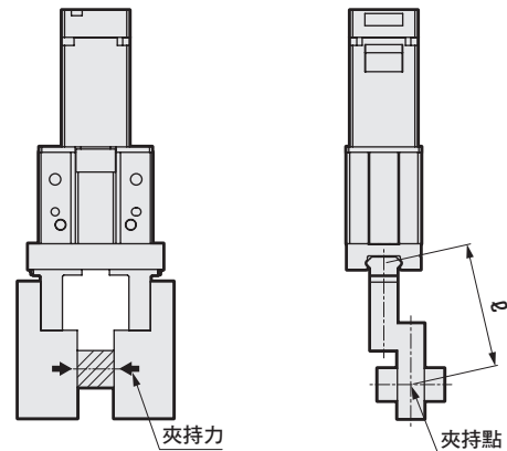
夾持力和夾持點距離 (例: FLSH-20)
