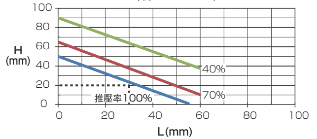
夾持點距離和推壓率 (例：FLSH-20)
