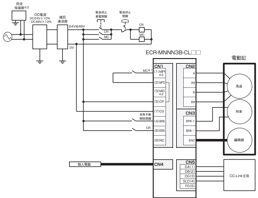
【CC-Link型】
