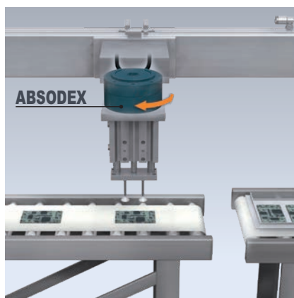
電子基板的搬運機
