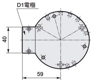
• 本體側 CHC-20R-D1
