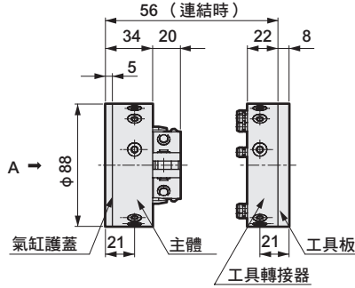
• 工具板圖
