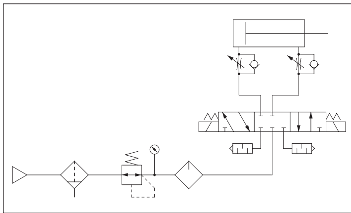
3位置中央封閉基本迴路圖
