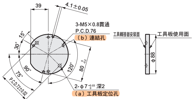
• 工具板圖
